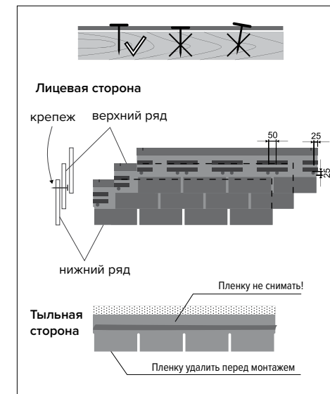
Рис. 1.1. Схема крепления фасадной плитки
